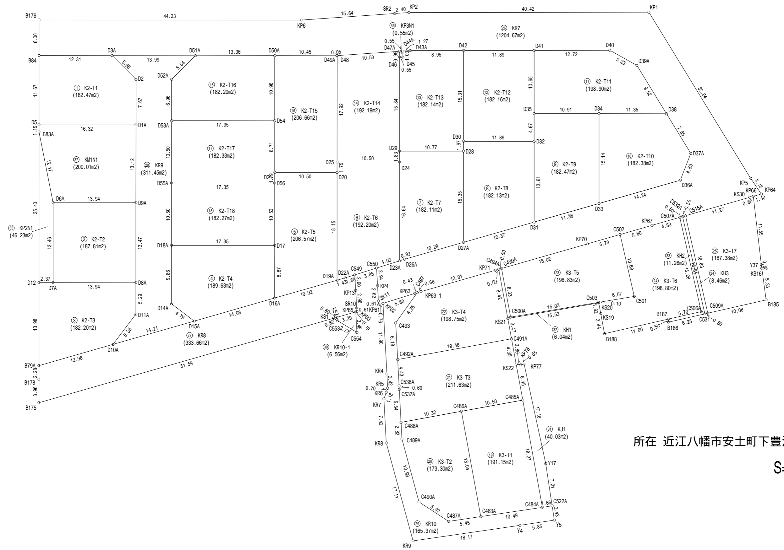
確定測量図 1
